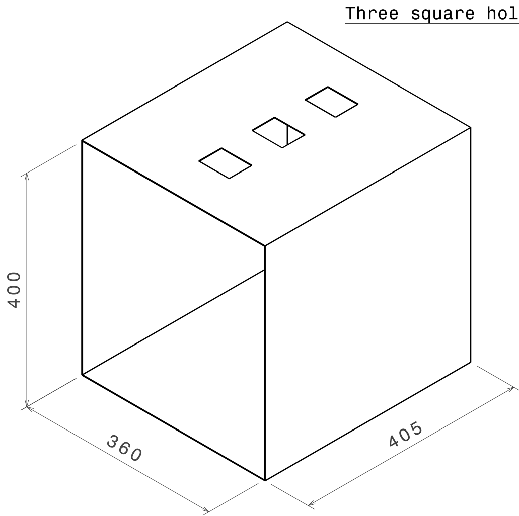
Isometric view Scale: 1:5
