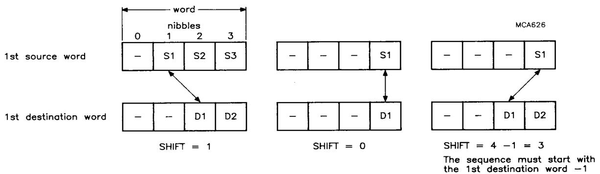
Fig.37 Shift example.
