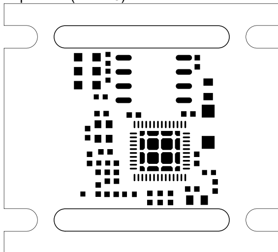
Top Paste (Scale 3)
