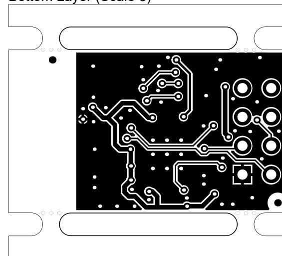
Bottom Layer (Scale 3)
