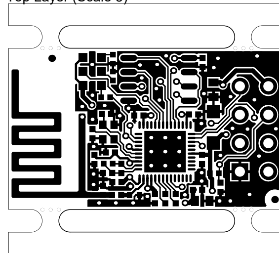
Top Layer (Scale 3)
