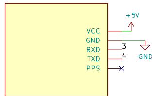
A1 GTU7GPSModule J1 GTU7GPSModule-Header-5POS
