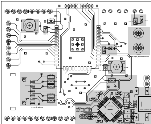
usb-uart bridge, optional
