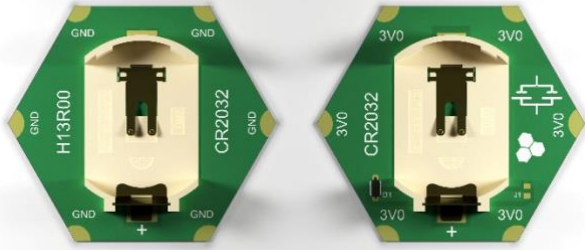
Bottom (1:1)
